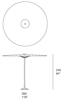
CA09C CA09D con snodo/ with joint con balze/with flounces
